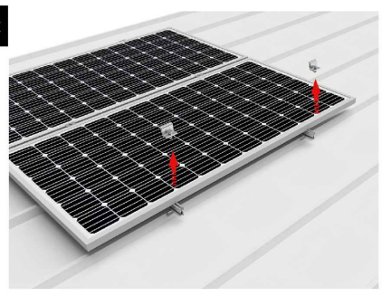
Kit 1 - Extraer presores laterales de los extremos a unir
