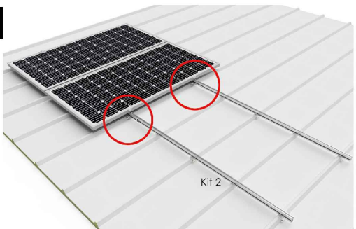
Kit 2 - Introducir los perfiles guía del Kit 2 en las uniones y fijar los perfiles del Kit 1 y 2 a las uniones con los tornillos de fijación
