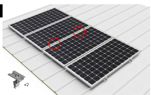
Kit 2 - Montar los módulos del Kit 2 y unir con los módulos existentes del Kit 1 mediante los presores centrales suministrados en el kit de unión.
