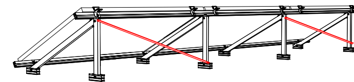
Arriostramiento ≥4 triángulos
