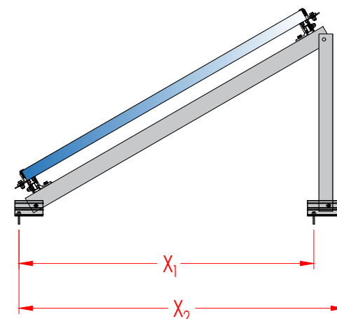
Arriostramiento 3 triángulos
